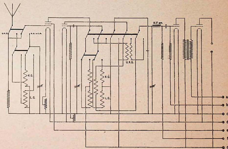
Fig. 1. Schakel-schema.
