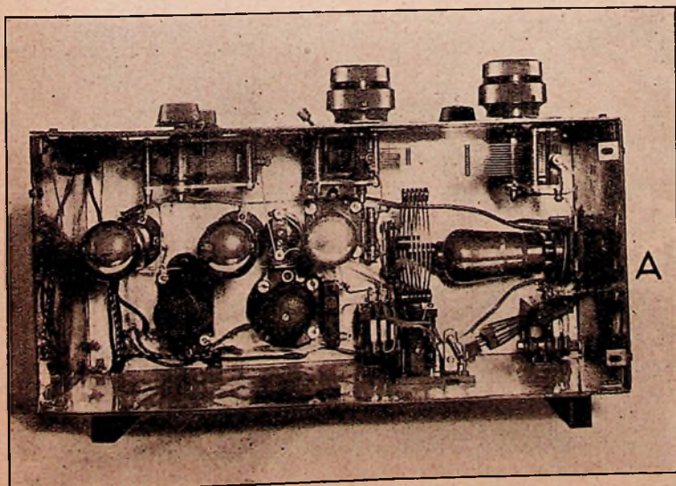
Bovenverdieping van het toestel, van bovengezien, met den completen ultra kortegolf-ontvanger.
