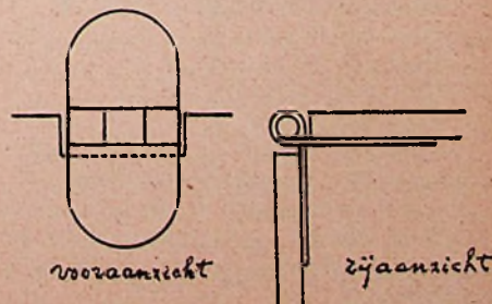
Fig. 2. Deksel-scharnier.
